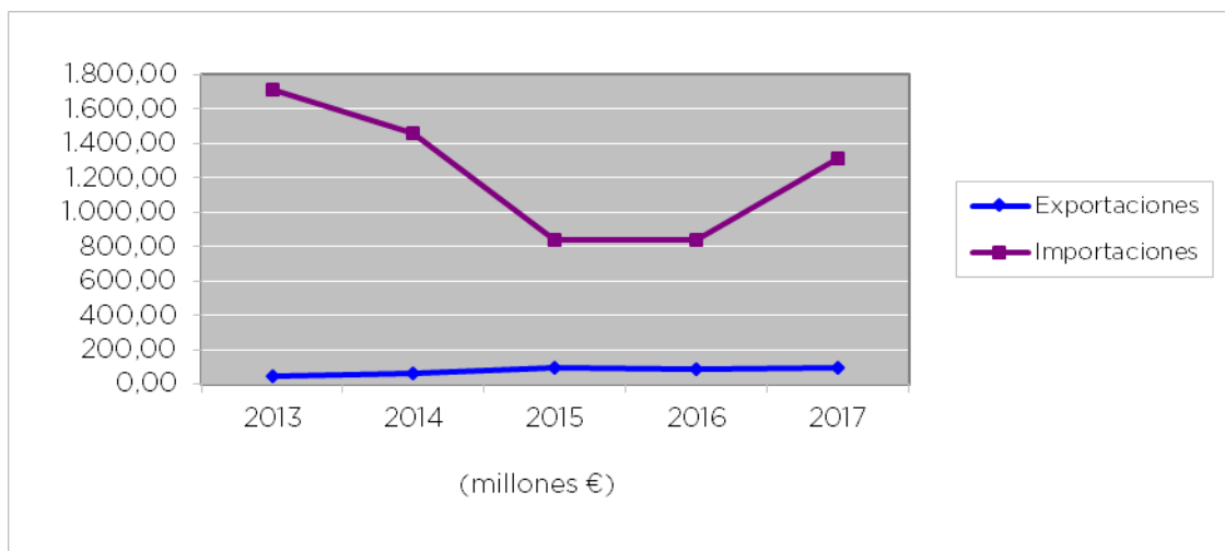
Gráfico 2. Evolución exportaciones Murcia-México. 2013-2017
